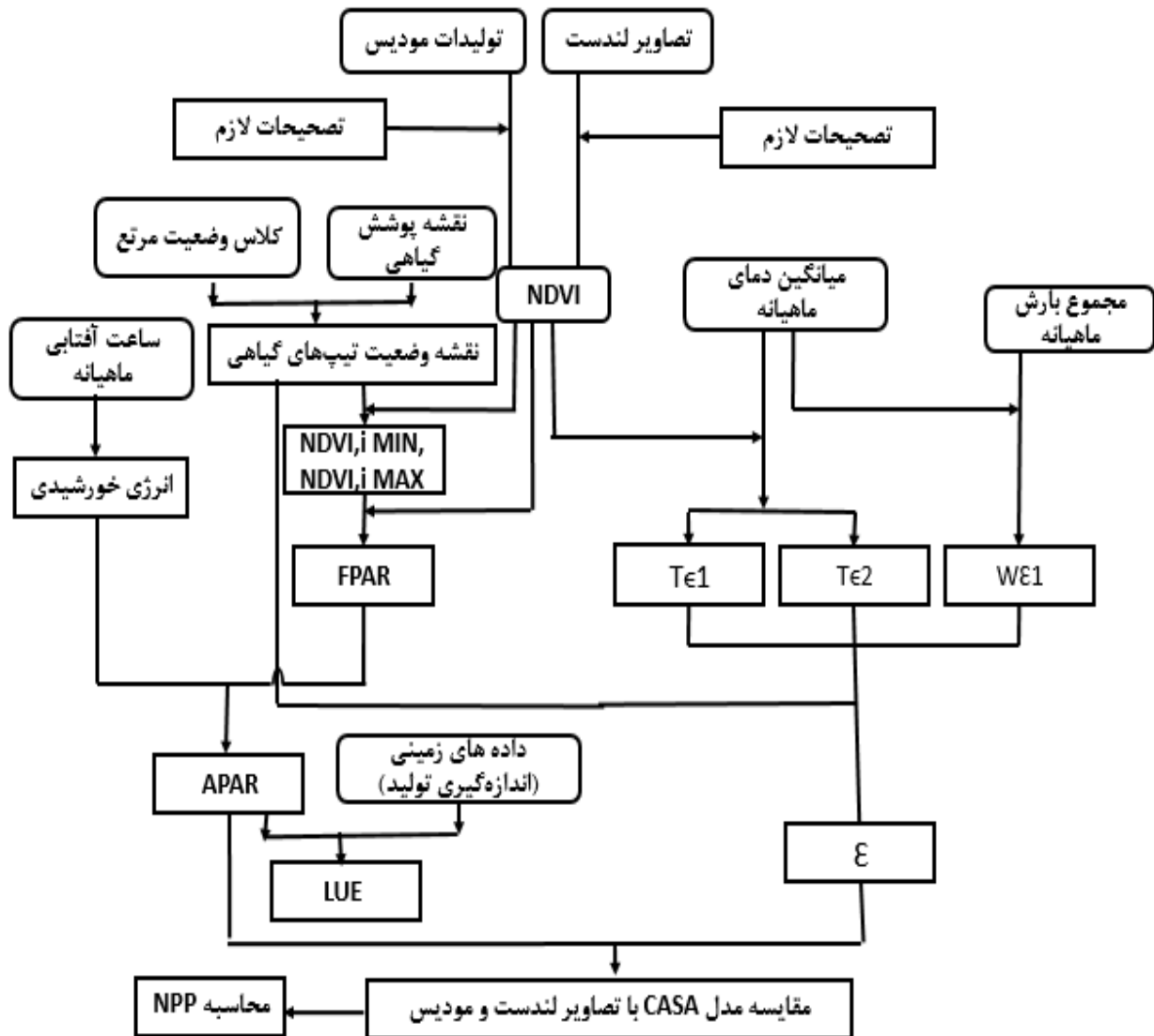
شکل ۲. نمودار گردش مراحل کار: NDVI_{i, MAX} و NDVI_{i, MIN} ؛ T\epsilon 1 ؛ T\epsilon 2 ؛ W\epsilon 1 ؛ FPAR ؛ APAR ؛ \epsilon ؛ LUE ؛ NPP محاسبه
