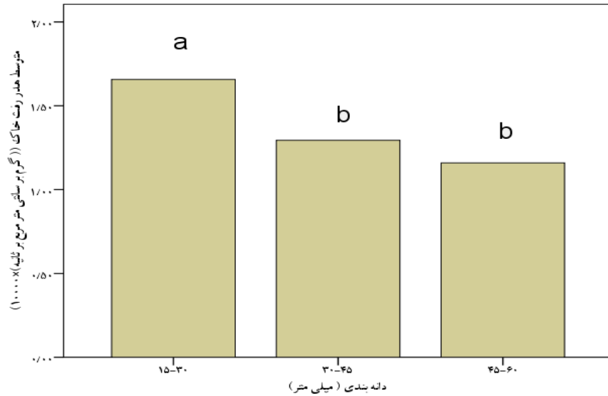
شکل ۶. اثر تیمار دانه‌بندی بر مقدار هدر رفت خاک
