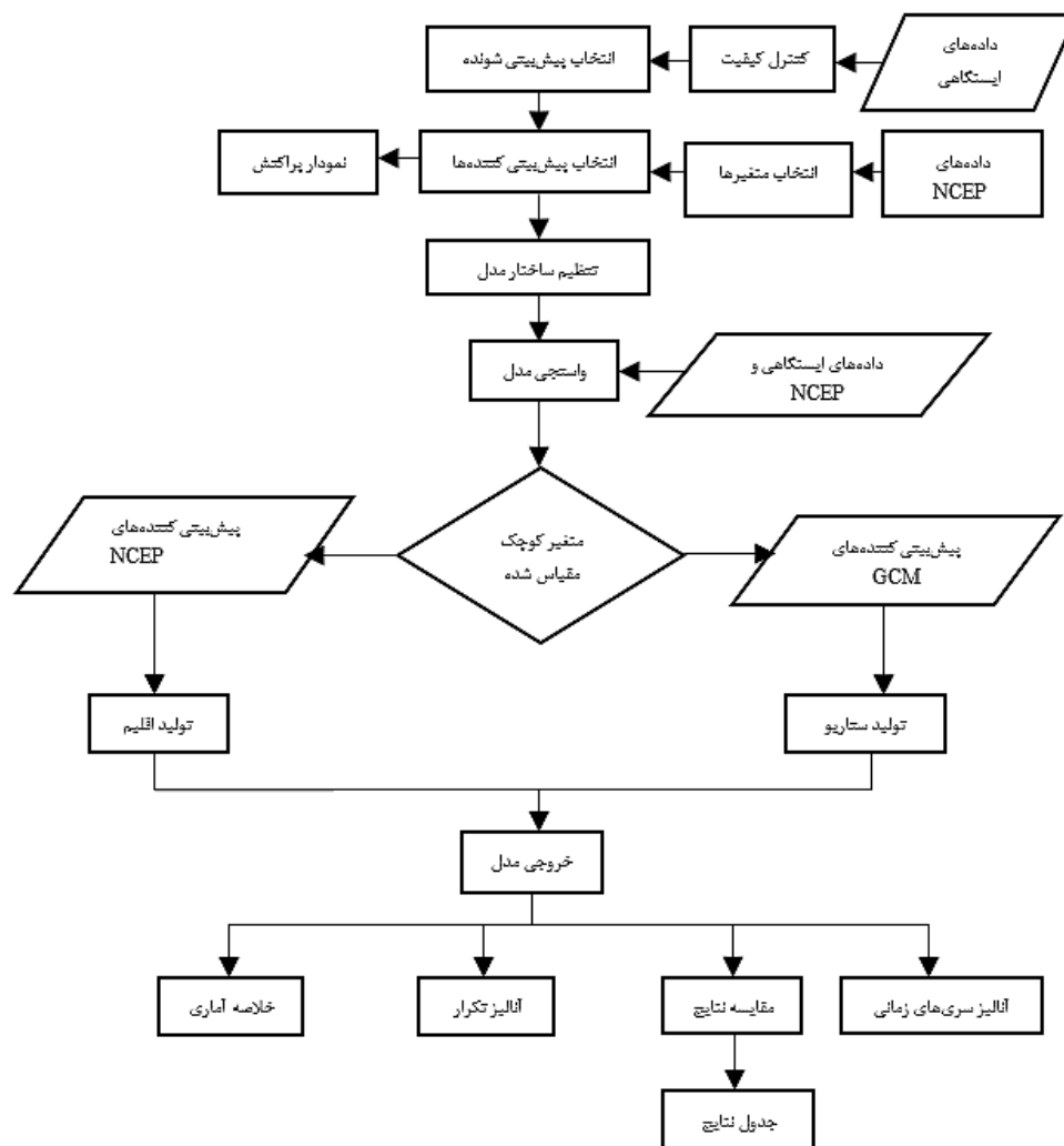
شکل ۲. مراحل کوچک مقیاس سازی آماری به روش SDSM (۱۲)
