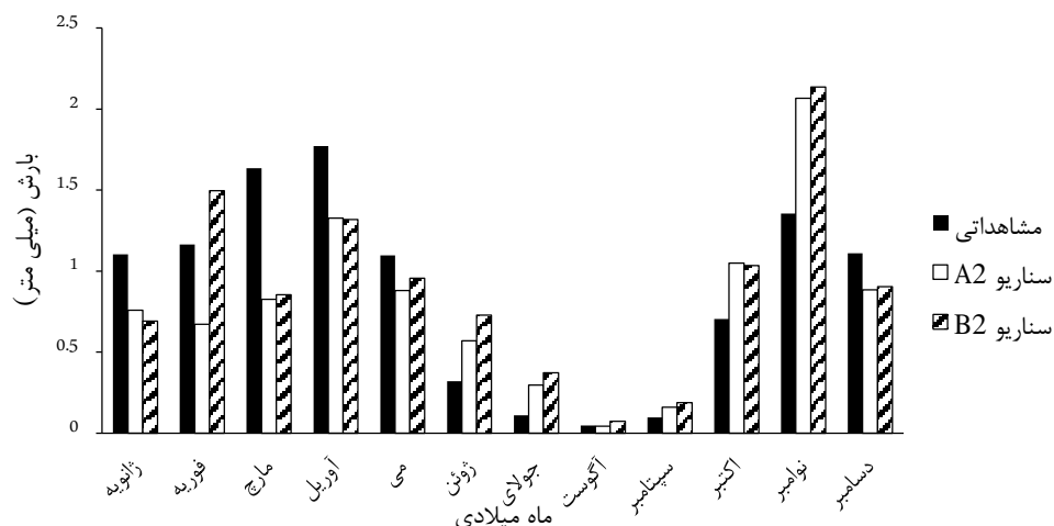
شکل ۱۱. میانگین بارندگی روزانه حوضه در دوره‌های مشاهده‌ای و سناریوسازی
