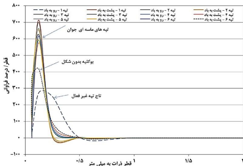
شکل 3. طبقه بندی تپه‌های ماسه‌ای بر اساس نمودار استاندارد با بنزر و بسلر
